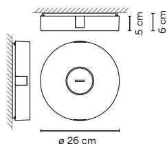
Surface Canopy M E2 Ø 260 mm.
